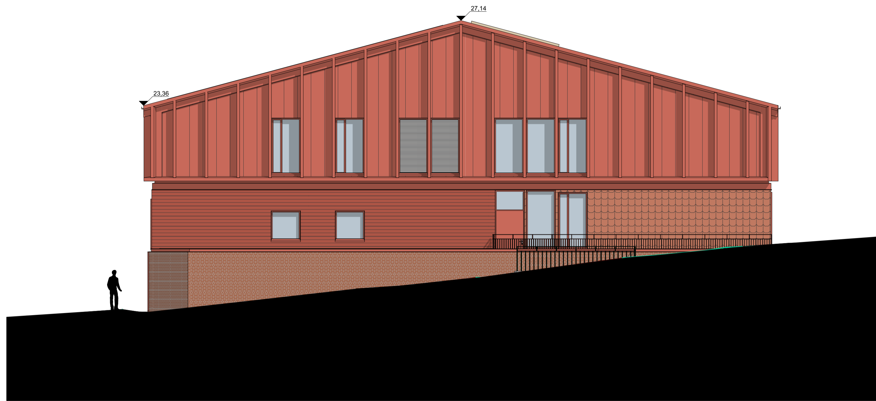
Fasade Øst
