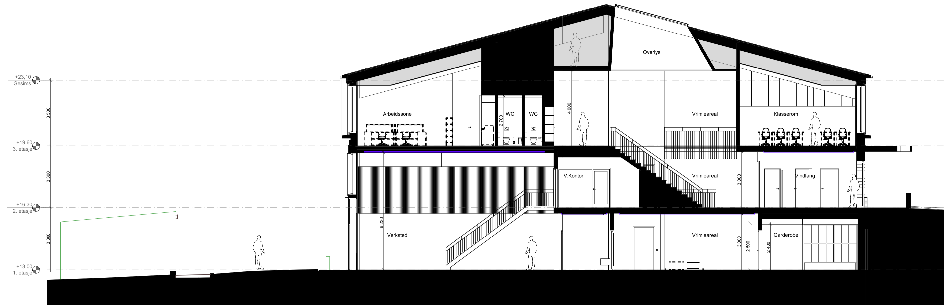
Snitt AA
