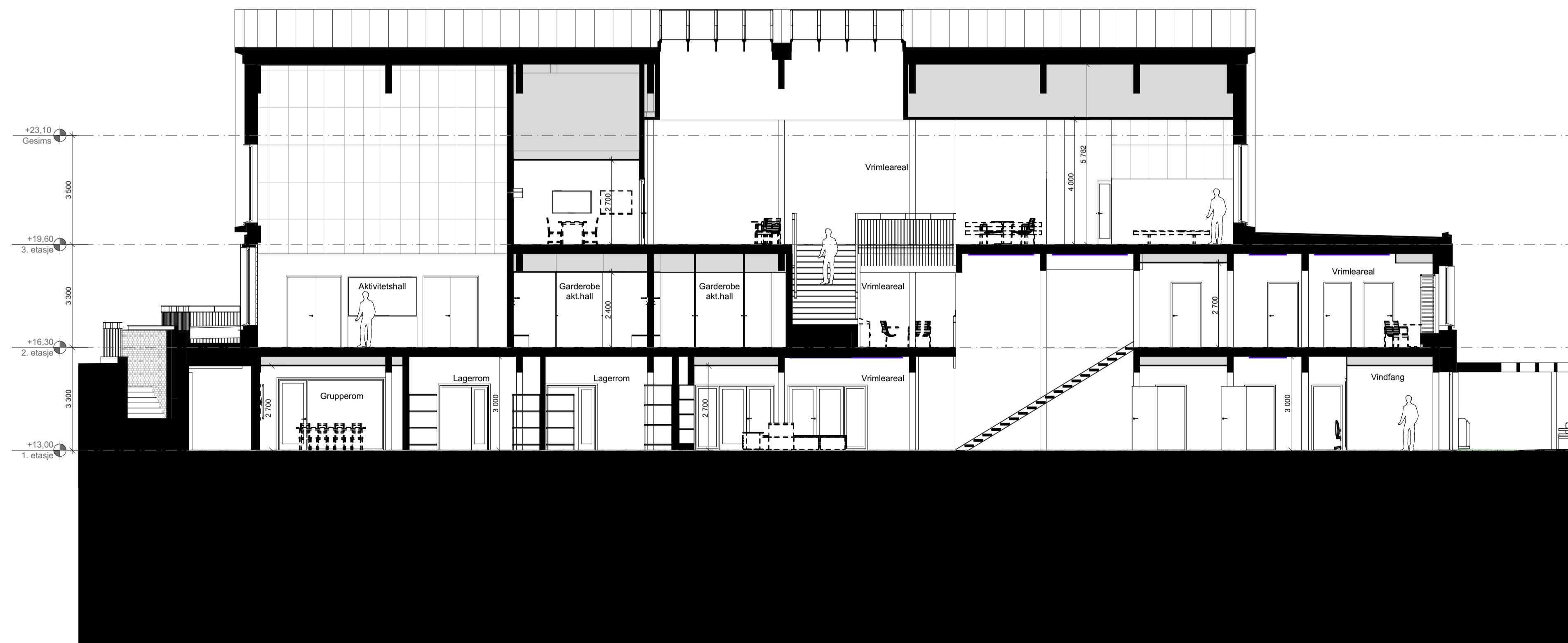
Snitt BB
